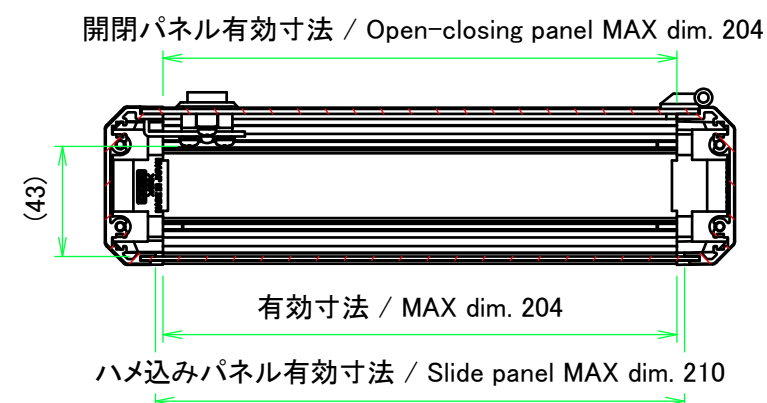
A-A (1:3)
