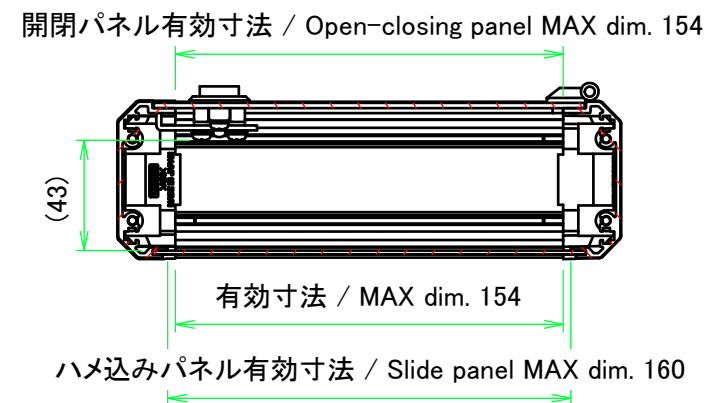
A-A (1:3)
