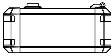
A-A (1:3)
