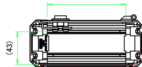
A-A (1:3)
