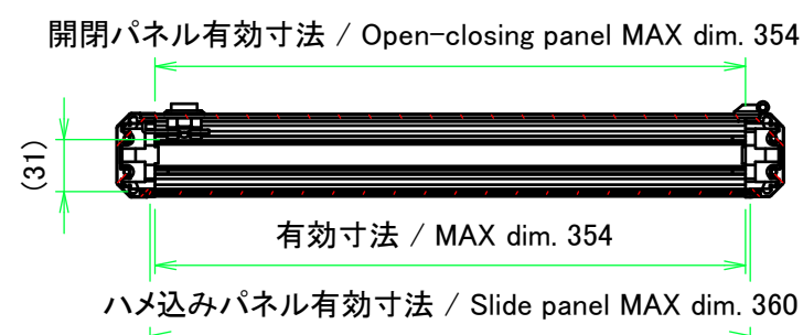
A-A (1:5)
