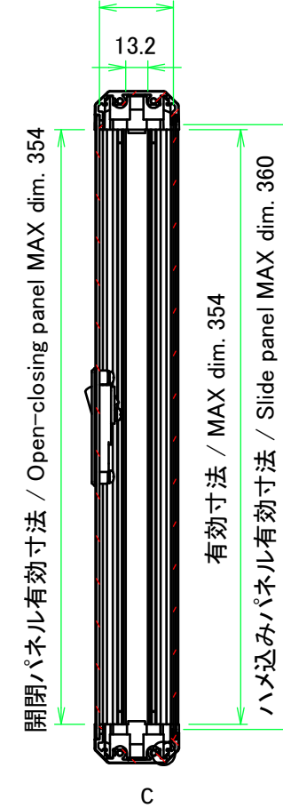
有効寸法 / MAX dim. 44
