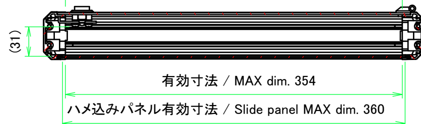
開閉パネル有効寸法 / Open-closing panel MAX dim. 354
