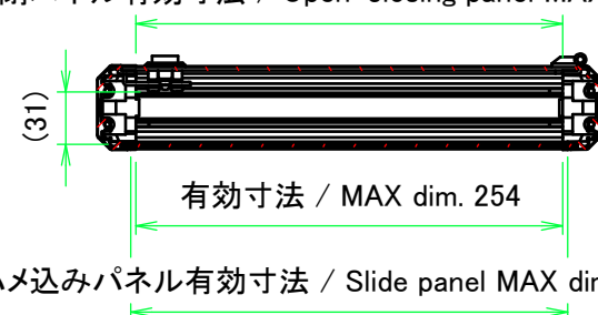
A-A (1:5)
