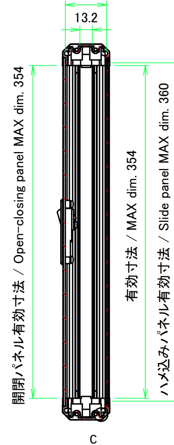
C: フレーム拡大図 / Frame cross-section
