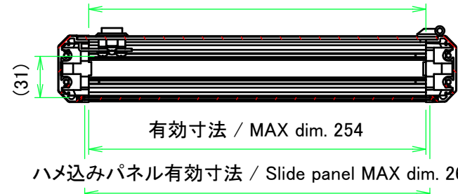
A-A (1:4)
