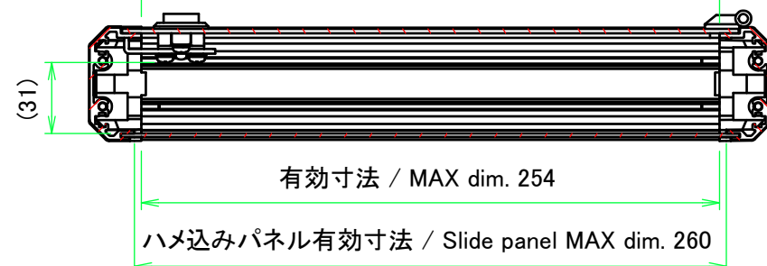
開閉パネル有効寸法 / Open-closing panel MAX dim. 254
