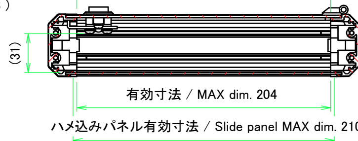
開閉パネル有効寸法 / Open-closing panel MAX dim. 204
