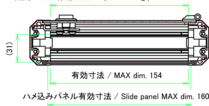
A-A (1:2.5)
