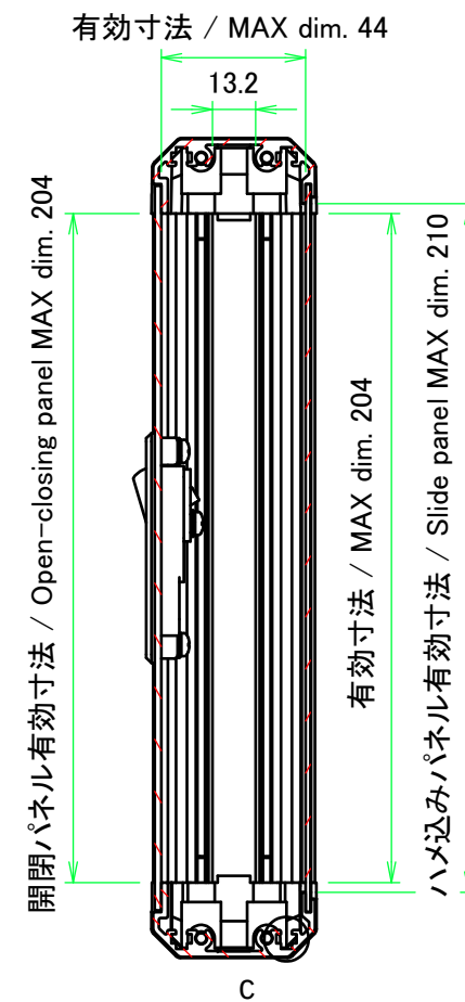
B-B (1:2.5)
