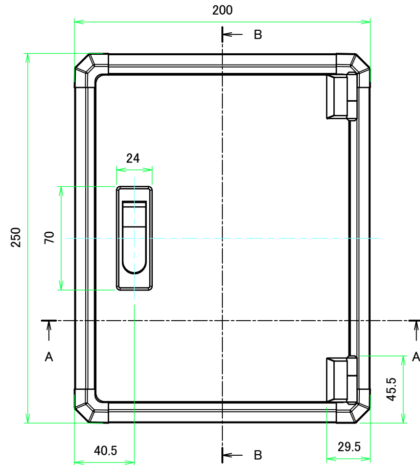
フレーム2側 / Frame2 side
