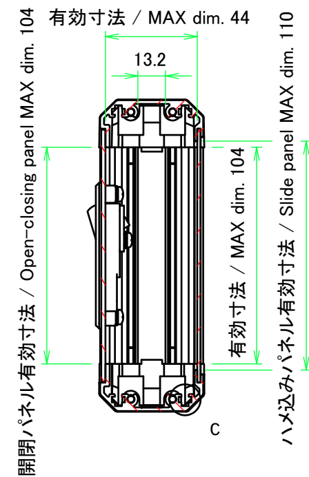
B-B ( 1 : 2.5 )
