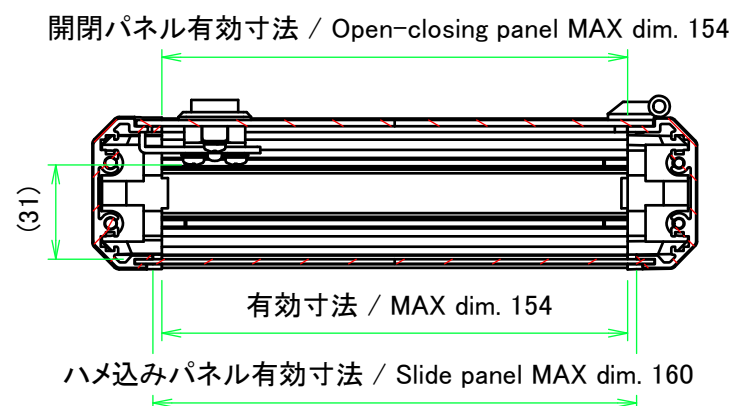
A-A ( 1 : 2.5 )
