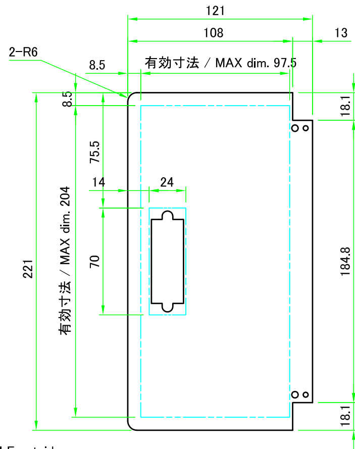
パネル表面/Panel Frontside
