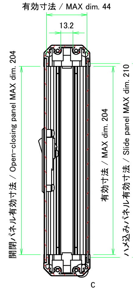
B-B ( 1 : 2.5 )
