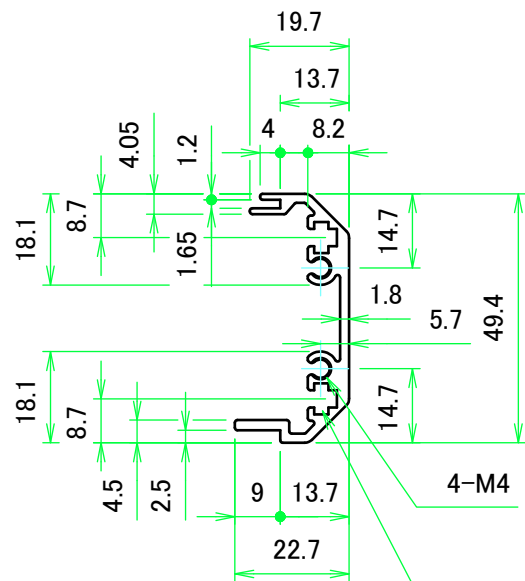
ナットレール / Nut rail
