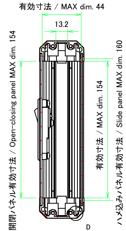
B-B ( 1 : 2.5 )
