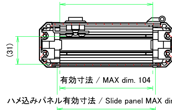
開閉パネル有効寸法 / Open-closing panel MAX dim. 104
