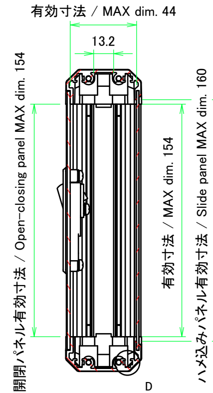
B-B ( 1 : 2.5 )
