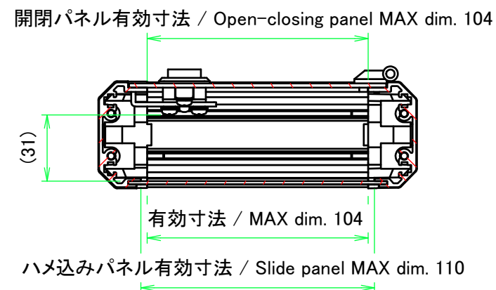
A-A ( 1 : 2.5 )
