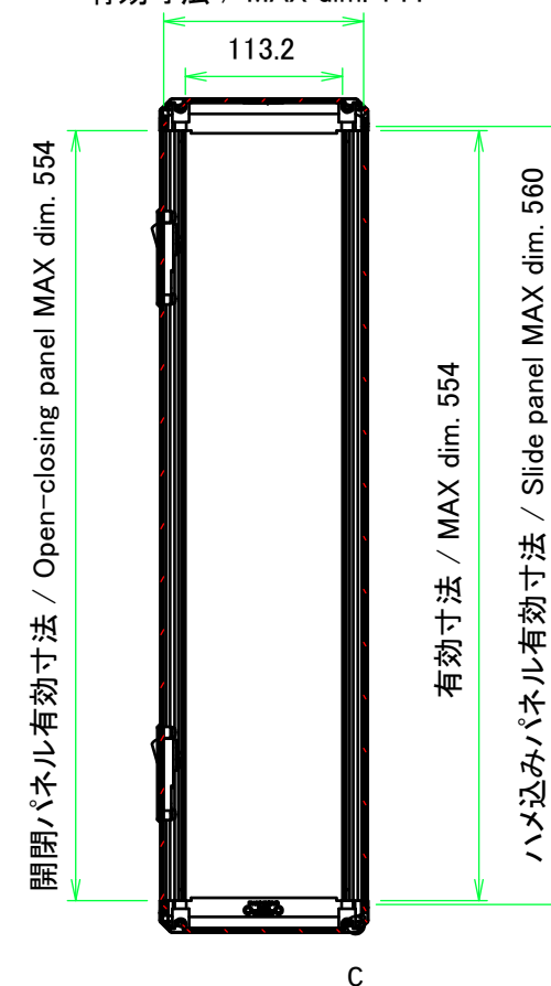
有効寸法 / MAX dim. 144
