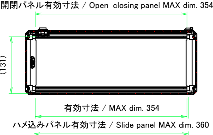
A-A ( 1 : 5.5 )
