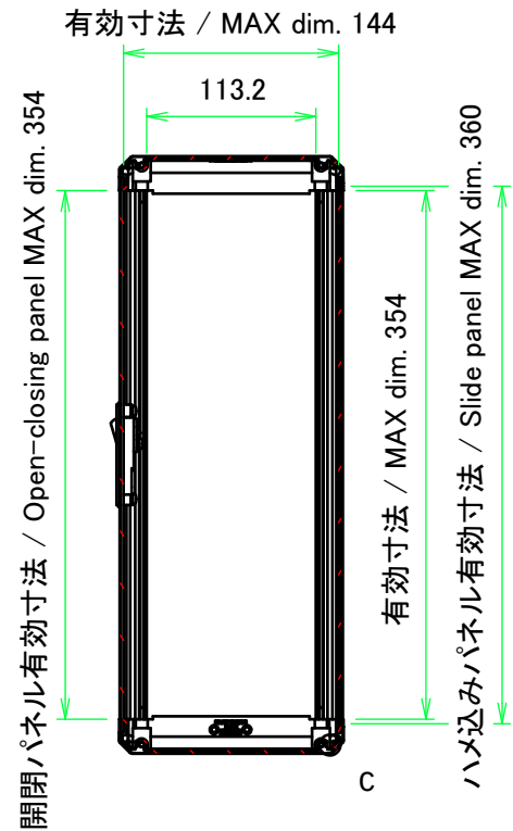
B-B ( 1 : 5.5 )
