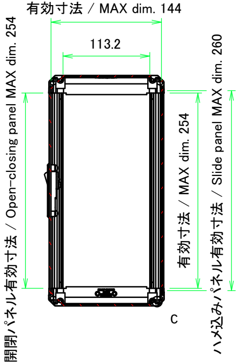
B-B ( 1 : 5 )
