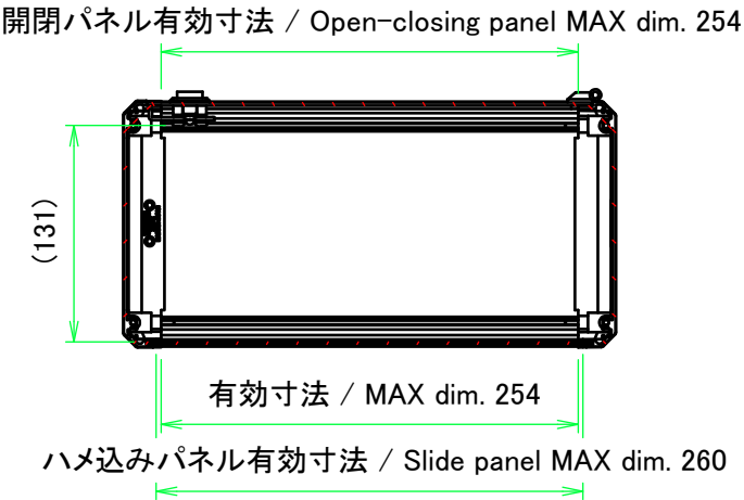
A-A ( 1 : 5 )
