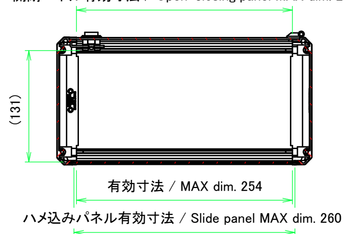
開閉パネル有効寸法 / Open-closing panel MAX dim. 254
