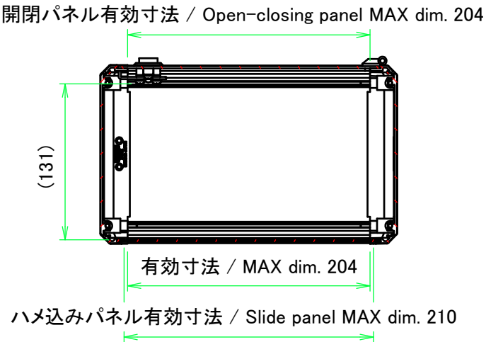
A-A ( 1 : 4.5 )
