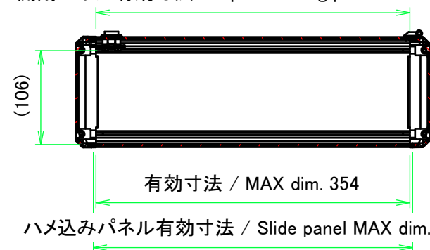
A-A (1:6)
