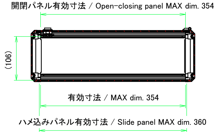
A-A ( 1 : 5.5 )
