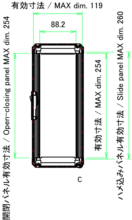
B-B ( 1 : 5.5 )
