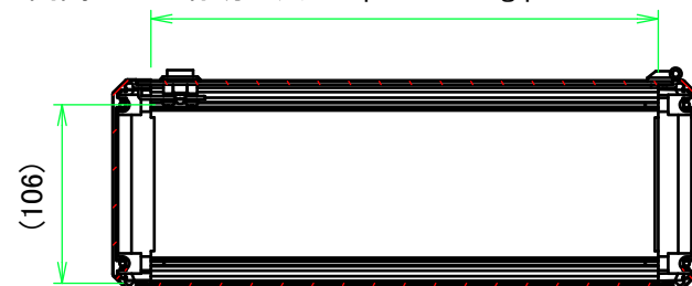
開閉パネル有効寸法 / Open-closing panel MAX dim. 304
