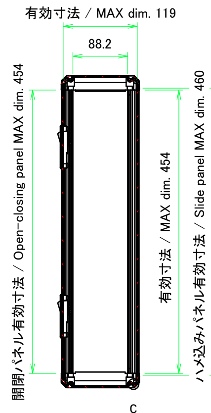
B-B ( 1 : 6 )
