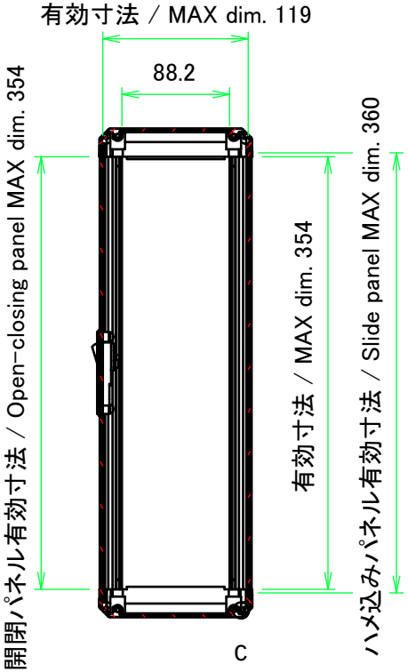
B-B ( 1 : 5.5 )
