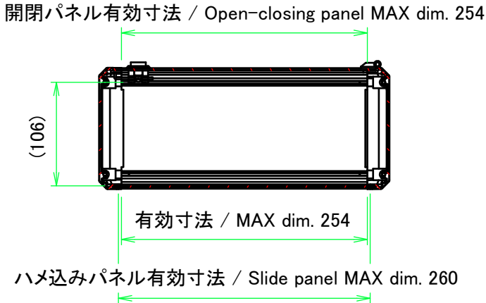
A-A ( 1 : 5.5 )
