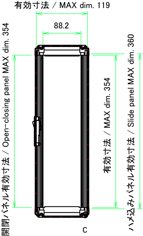
B-B ( 1 : 5.5 )
