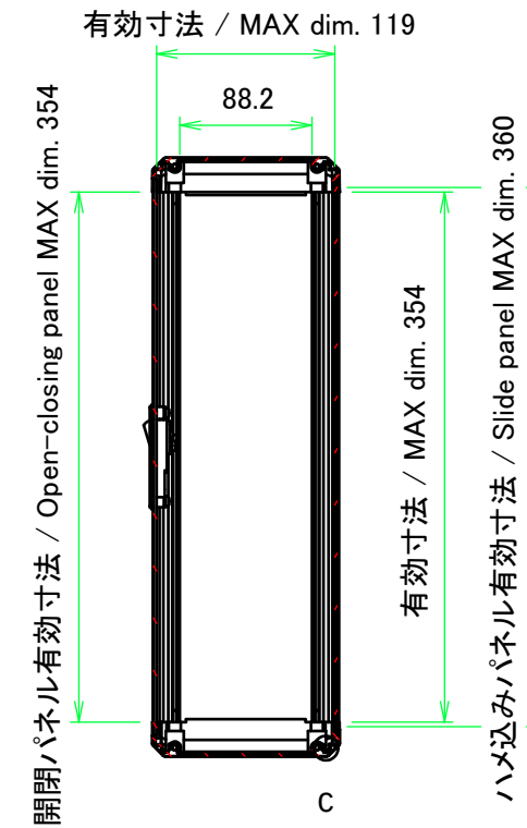
B-B ( 1 : 5.5 )
