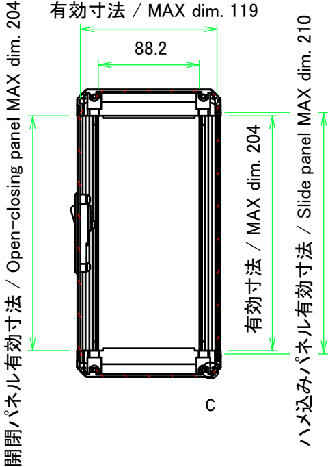
B-B ( 1 : 4.5 )
