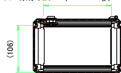
A-A ( 1 : 5 )
