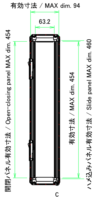
B-B ( 1 : 6 )
