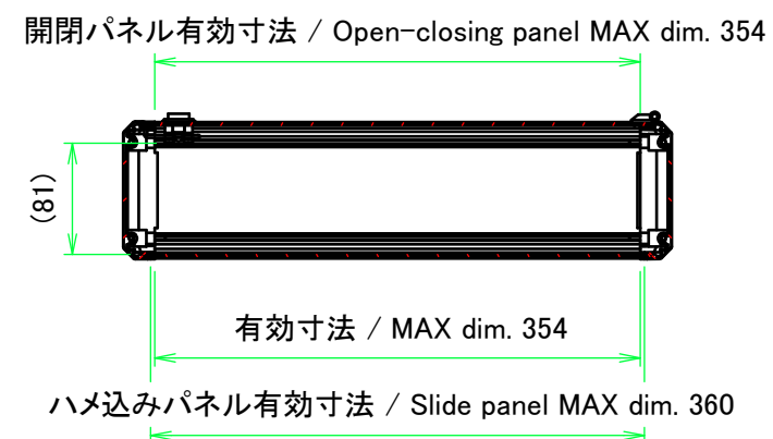
A-A ( 1 : 6 )
