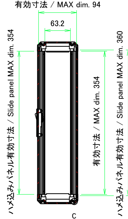
B-B ( 1 : 5.5 )
