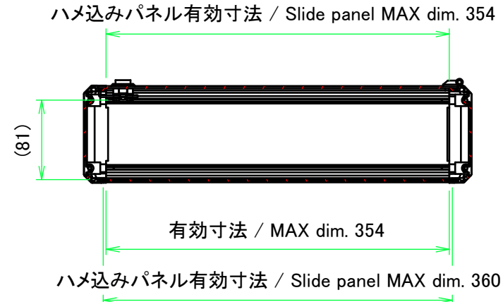
A-A ( 1 : 5.5 )
