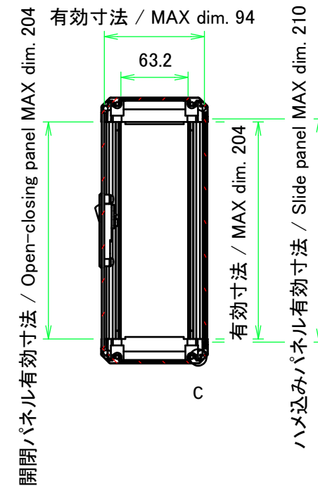
B-B ( 1 : 5 )
