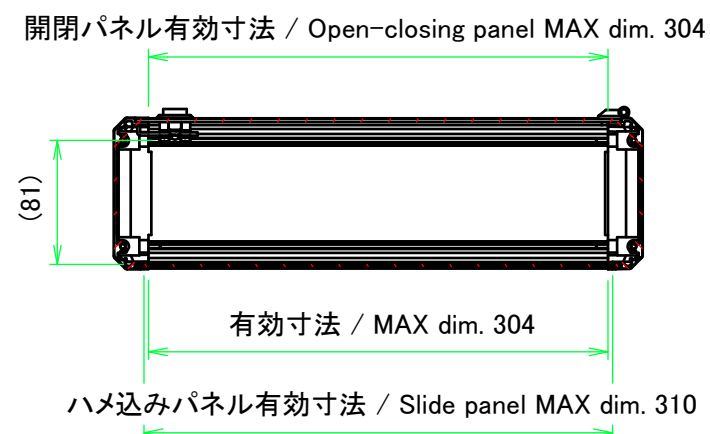
A-A ( 1 : 5 )
