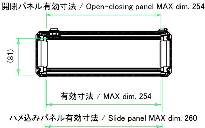
A-A (1:5)
