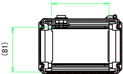
A-A ( 1 : 4 )
