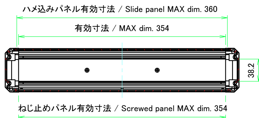
A-A ( 1 : 4 )
