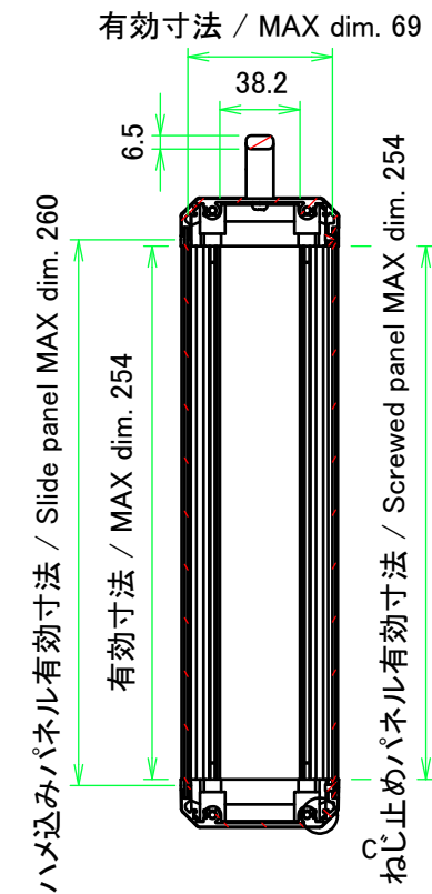
B-B ( 1 : 4 )
