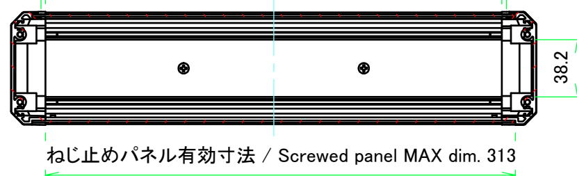
有効寸法 / MAX dim. 304
