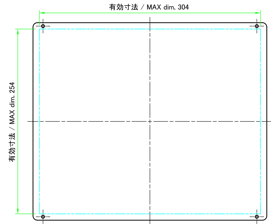
パネル表面/Panel Frontside
