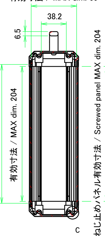
有効寸法 / MAX dim. 69
