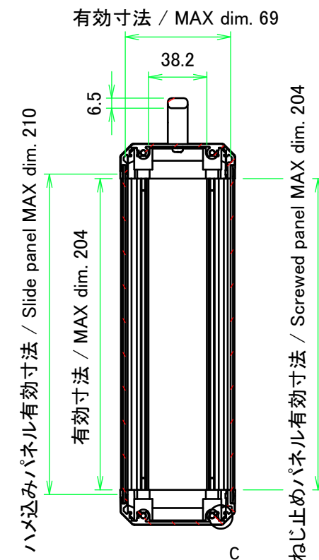
B-B ( 1 : 3.5 )
