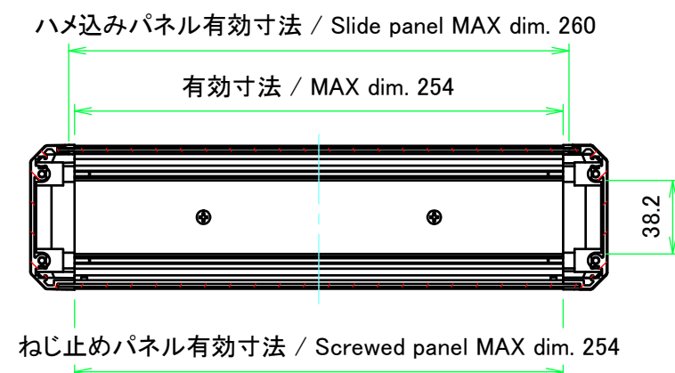
A-A ( 1 : 3.5 )
