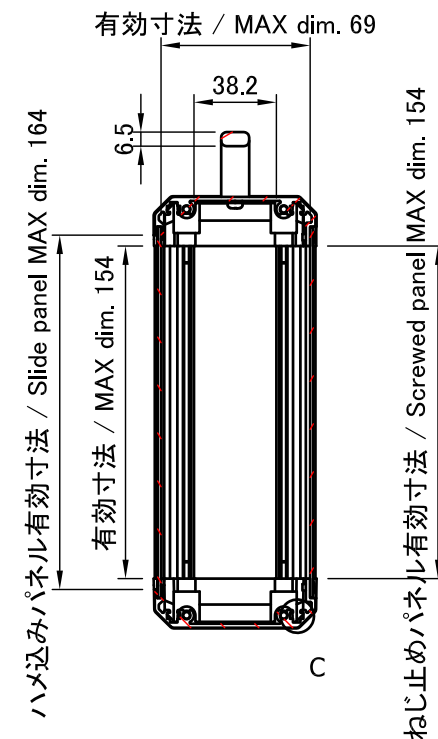
B-B (1:3.5)
