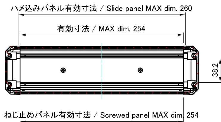
A-A (1:3.5)
