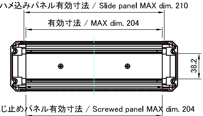
A-A (1:3.5)
