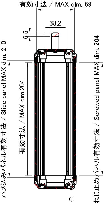
B-B (1:3.5)
