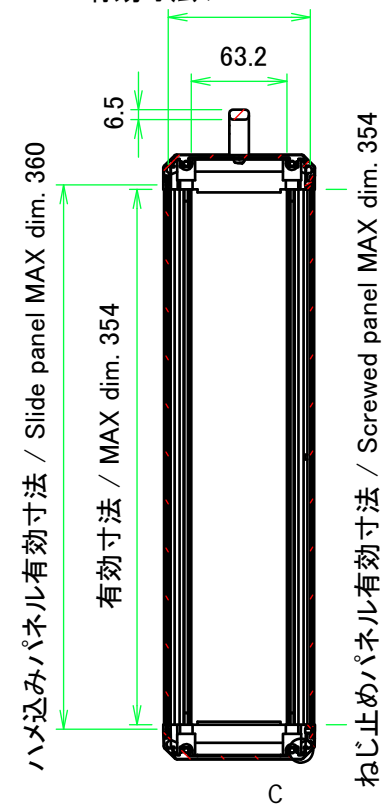
有効寸法 / MAX dim. 94
