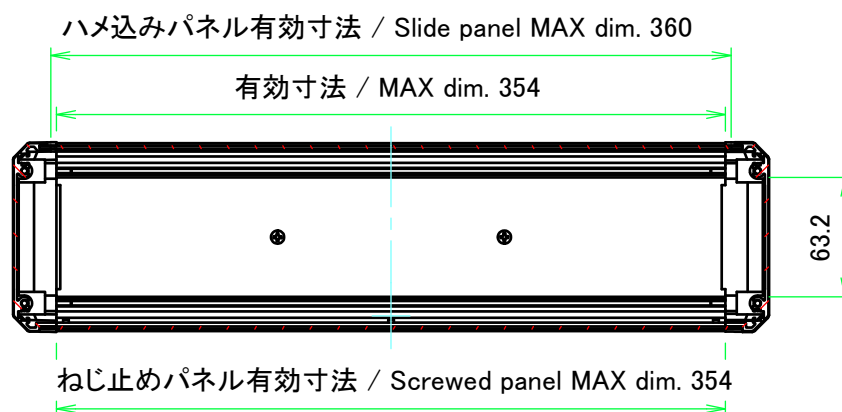
A-A (1:4)
