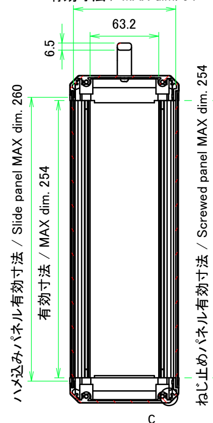
有効寸法 / MAX dim. 94
