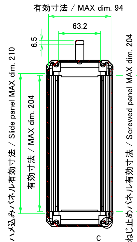
B-B (1:3.5)
