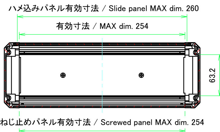
A-A ( 1 : 3.5 )
