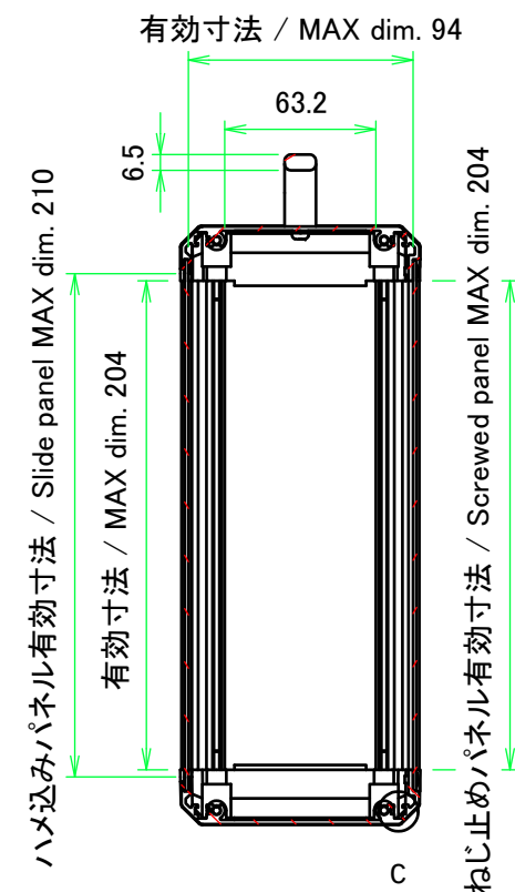
B-B ( 1 : 3.5 )
