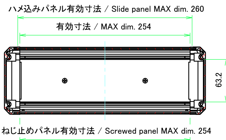
A-A (1 : 3.5)
