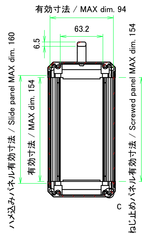
B-B (1 : 3.5)
